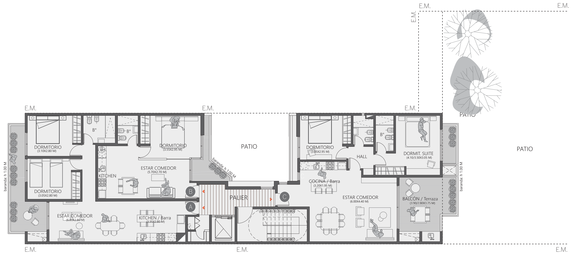
Planta piso 7°
