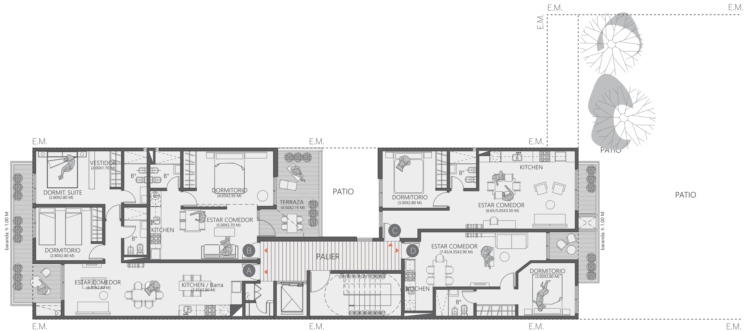
Planta piso 1°
