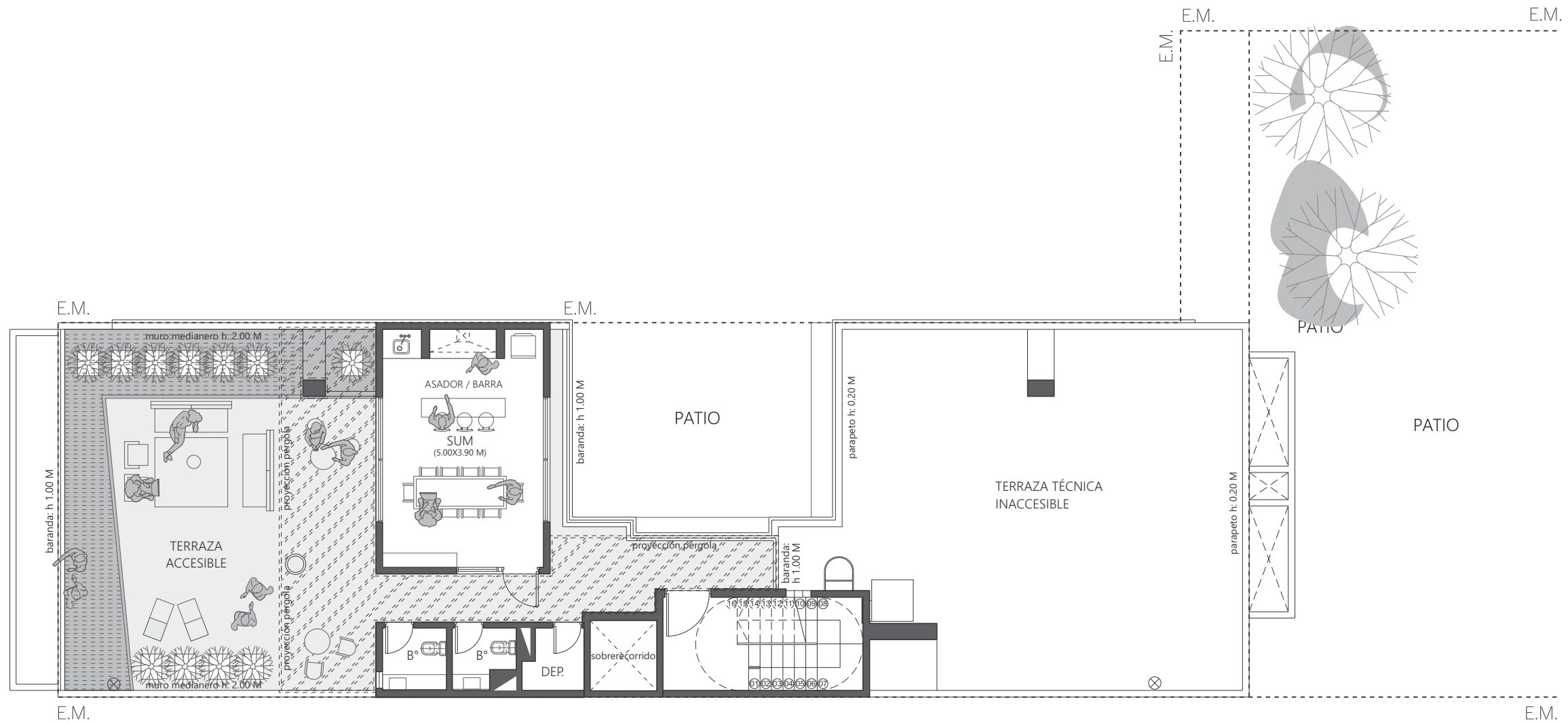
Planta piso 8°
